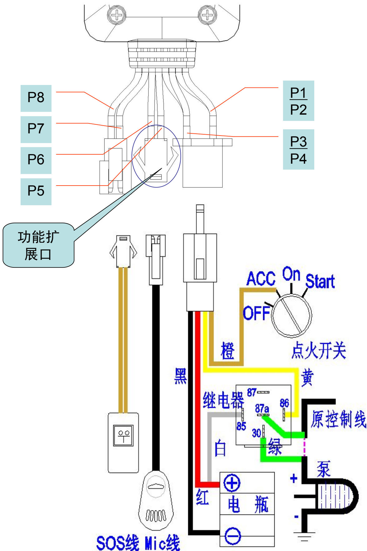
外接管脚定义总图
